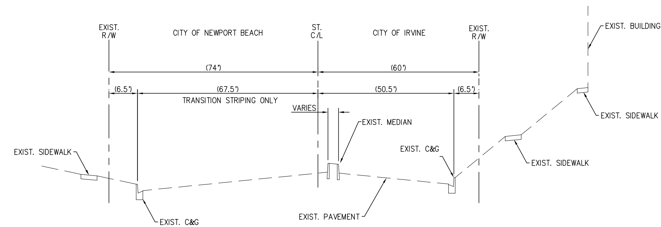
SECTION E-E N.T.S.
